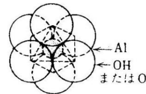
図 3.1 層状ケイ酸塩鉱物の基本構造 (三枝, 1989)
