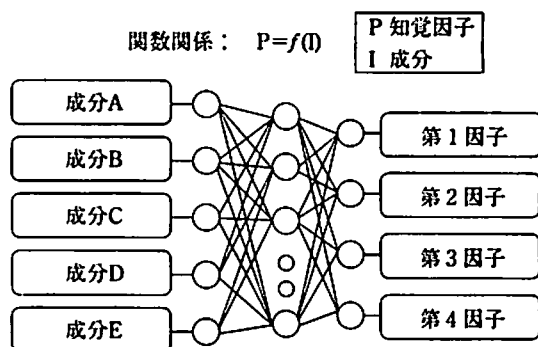
図3 ANNモデルの構造
