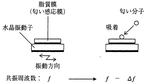
図8 水晶振動子式匂いセンサの構造と原理 (1)
