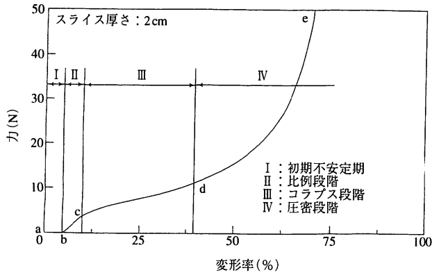
図13 食パンクラムの圧縮力-変形率曲線
